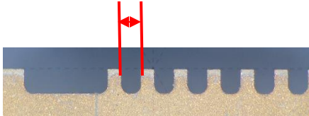
細線ワイヤー径0.05により幅0.1角R0.05加工が可能
