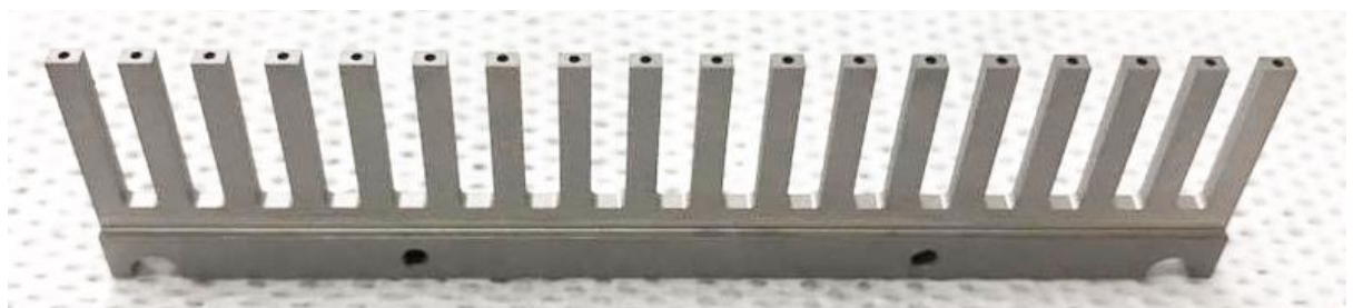
φ0.3電極により板厚20mmに18ヶ所 ワイヤ仕上がりφ0.7
