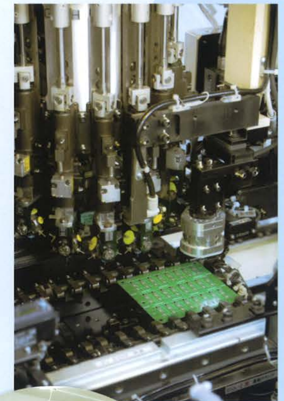
チップマウンター
