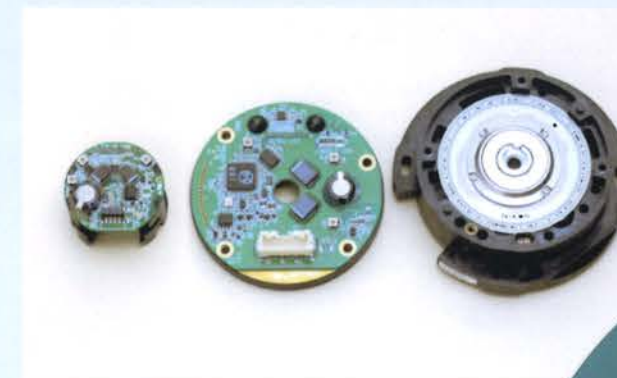
エンコーダー実装
