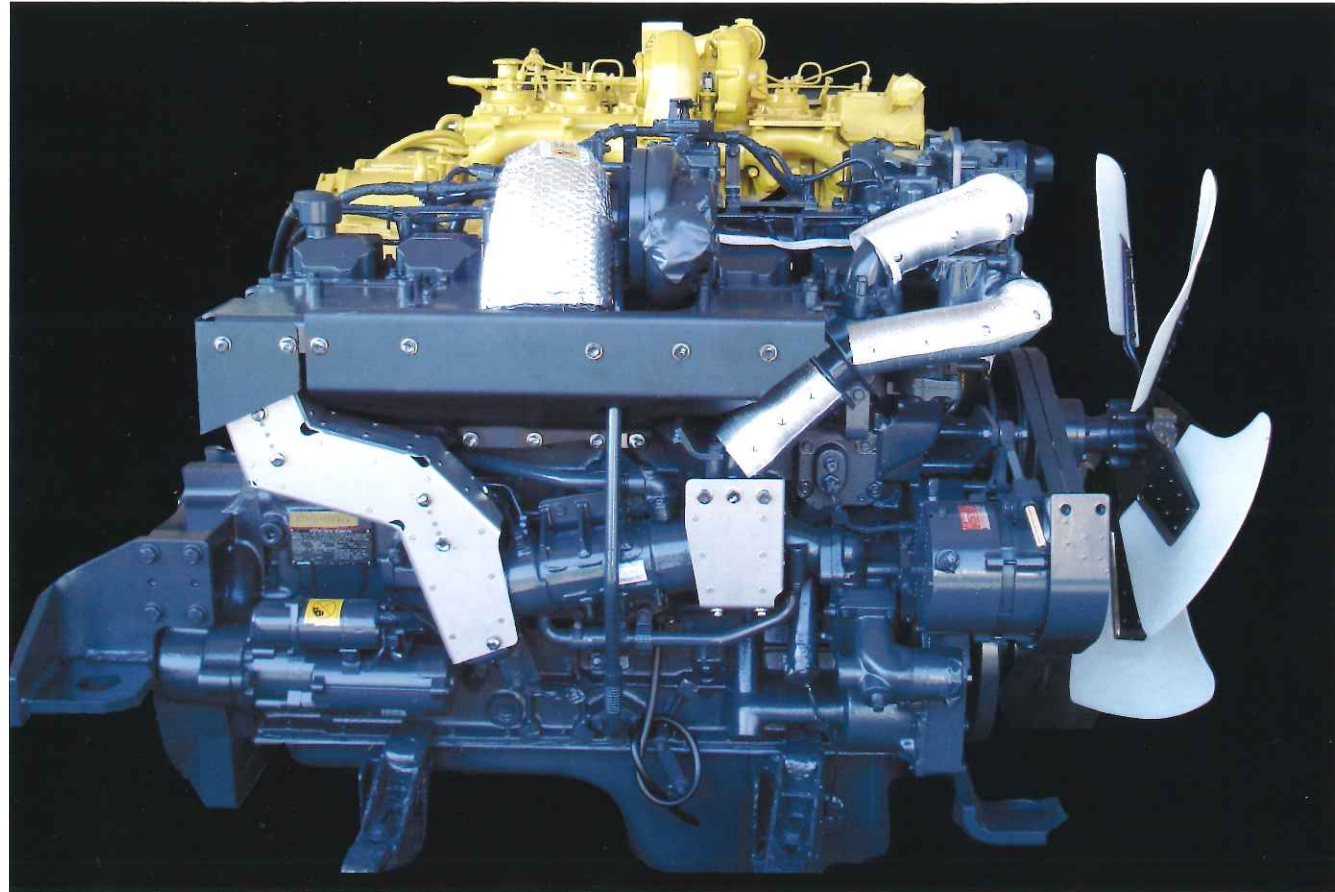
遮熱カバーエンジン取付・実例 Example: Installed Heat Insulators
